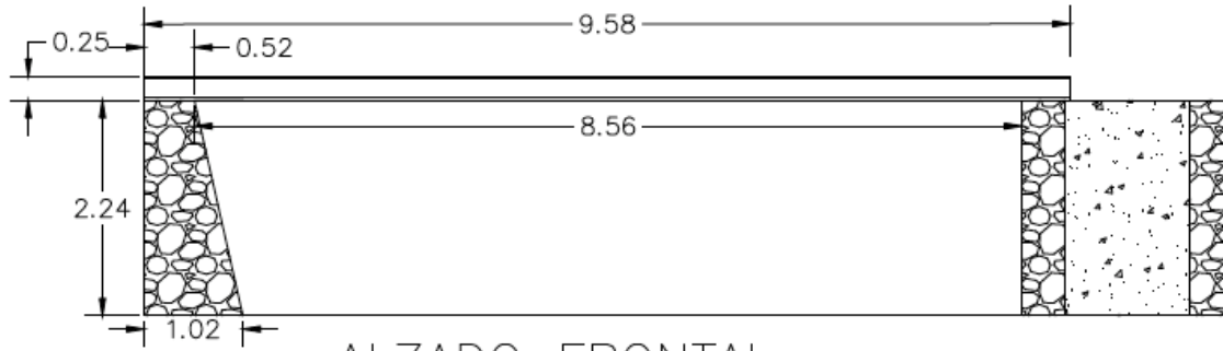
ALZADO FRONTAL
