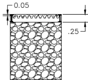
CORTE LATERAL
