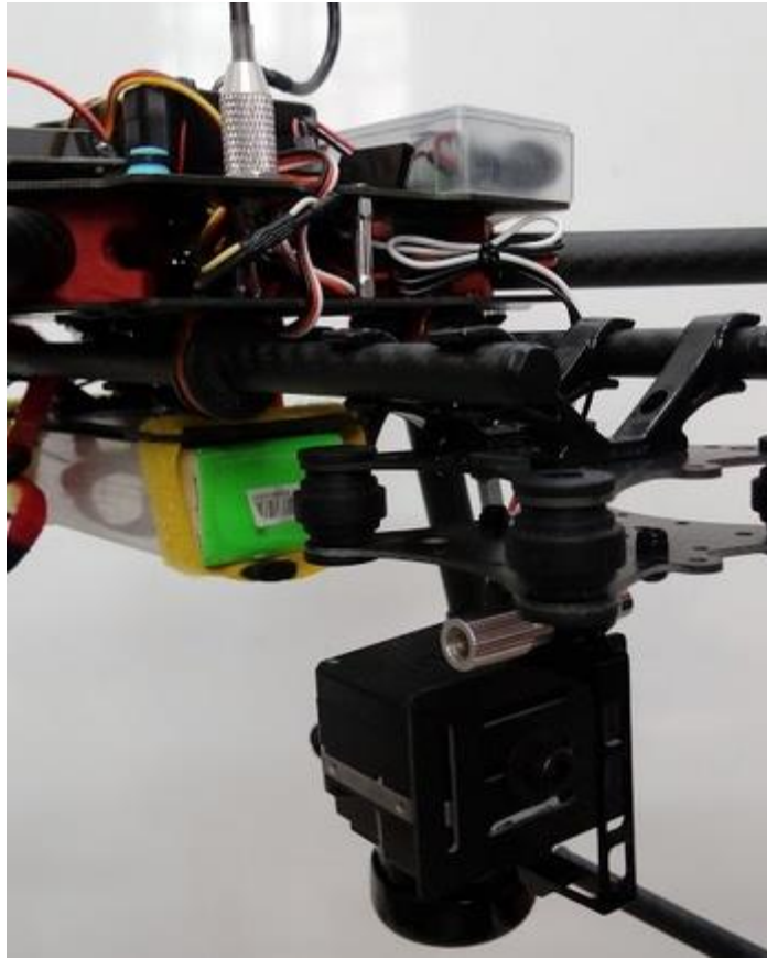
Figura 3.1: Acoplamiento mecánico de la cámara térmica, el regulador y cables conectores (fuente de la imagen: propia).
