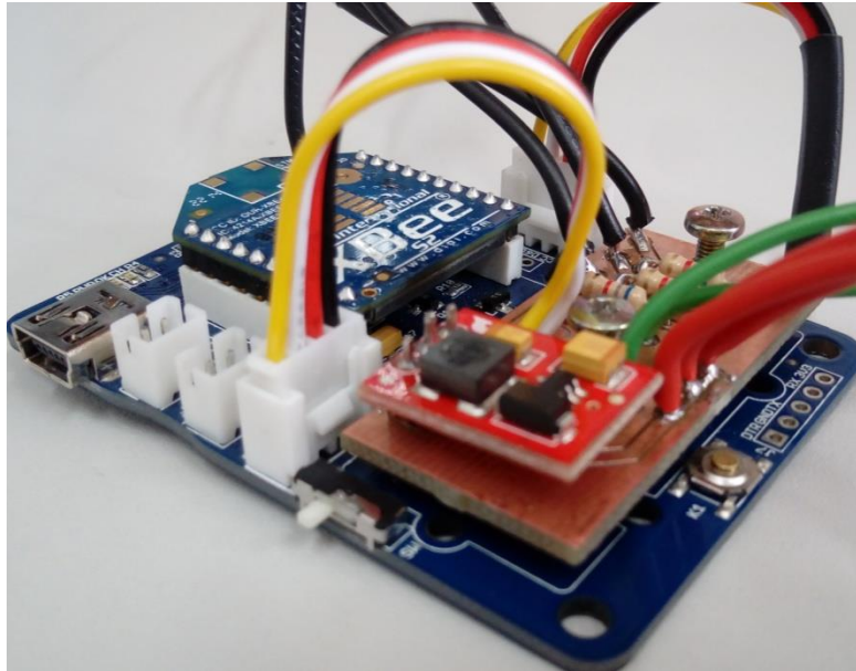
Figura 3.2: Acoplamiento en la tarjeta Grove-XBee Carrier del PCB que contiene al módulo SparkFun de 3.3V a 5V (fuente de la imagen: propia).
