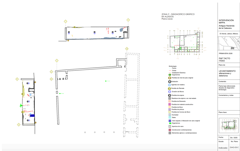
Plano de Zona C con alzados de estudio (sin escala)
