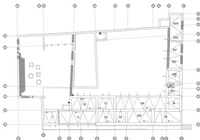
Plano de Azotea con Cuadrante Crítico señalado. Plano 2.
