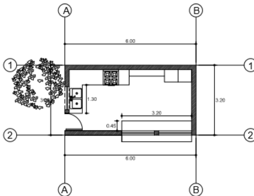
PLANTA ARQUITECTÓNICA
