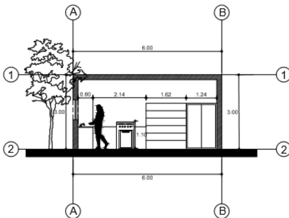
CORTE LONGITUDINAL
