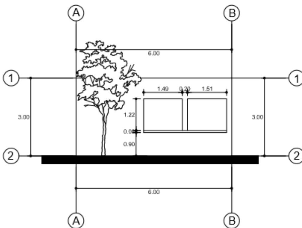
ALZADO FRONTAL
