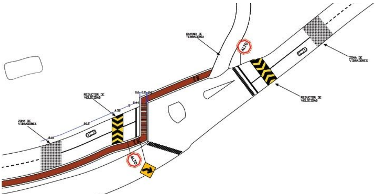
Imagen no. 118: Diagrama en cad de solución para cruce 1: salida de Atotonilco el Alto. Desarrollado durante el periodo Otoño 2020.
