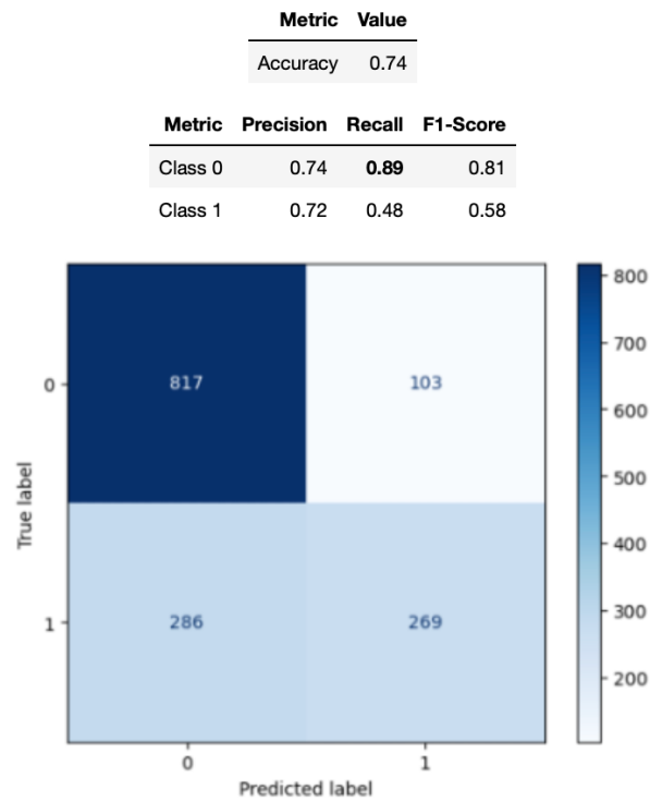
Figura 29. Métricas Bagging con GBC Test
