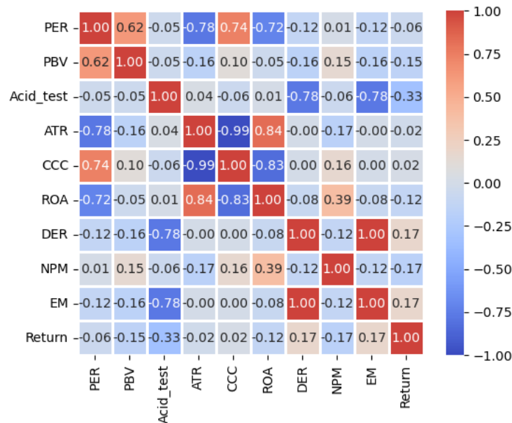
Figura 19. Análisis de correlación Spearman
