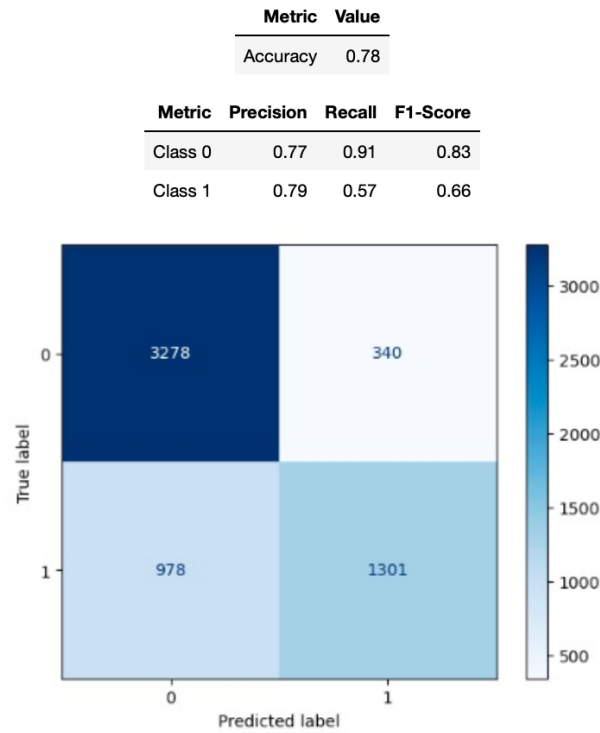
Figura 28. Métricas Bagging con GBC Train
