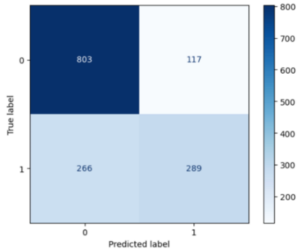
Figura 27. Métricas GBC Test
