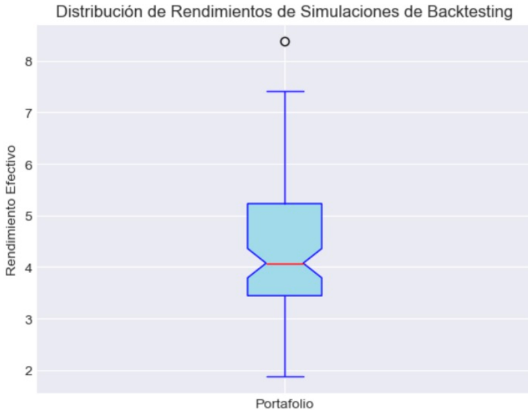
Figura 46. Gráfica Boxplot de Distribución de Rendimientos en Efectivo.
