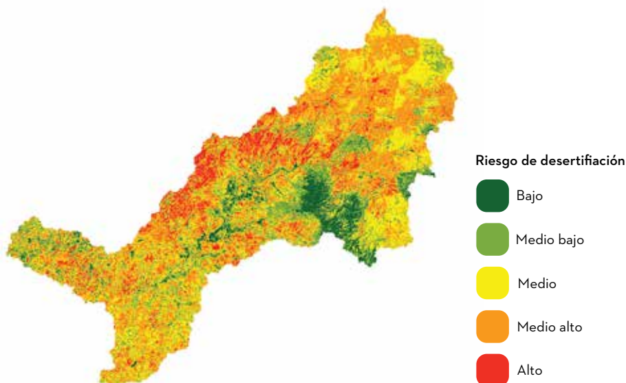
FIGURA 9.10 RIESGO DE DESERTIFICACIÓN PARA LA CUENCA DEL RÍO LAGOS
