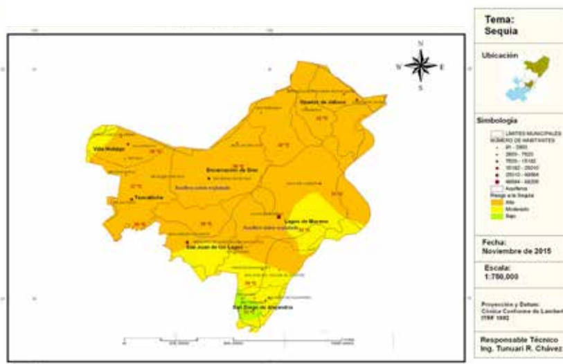
FIGURA 3.7 RIESGO DE SEQUÍA EN EL ÁREA DE ESTUDIO
