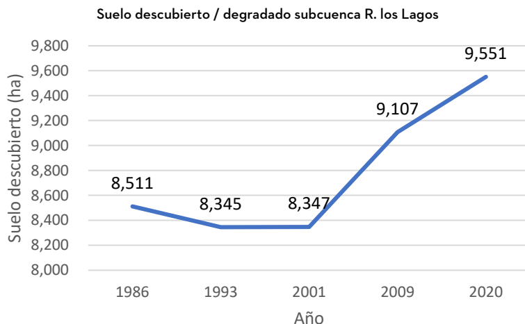
FIGURA 9.7 EVOLUCIÓN DE LA SUPERFICIE DE SUELO DESCUBIERTO EN LA SUBCUENCA DEL RÍO LAGOS, 1986-2020
