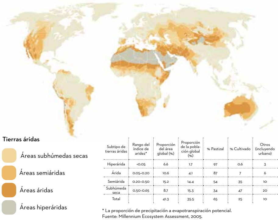
FIGURA 1.1 DISTRIBUCIÓN GEOGRÁFICA DE TIPOS DE TIERRAS ÁRIDAS POR ÍNDICE DE ARIDEZ
