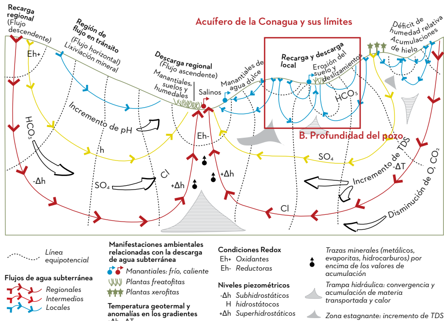
FIGURA 2.5 DIAGRAMA DE ELEMENTOS DE LOS SISTEMAS DE FLUJO DE AGUA SUBTERRÁNEA Y SUS CONDICIONES DE CONTROL
