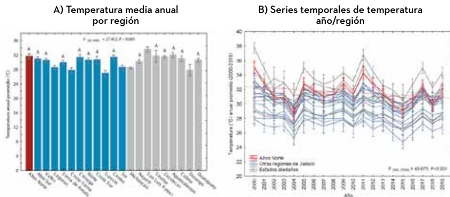
FIGURA 8.4 TEMPERATURA MEDIA ANUAL HISTÓRICA EN ALTOS NORTE Y SUS REGIONES DE INFLUENCIA, 2000-2019
