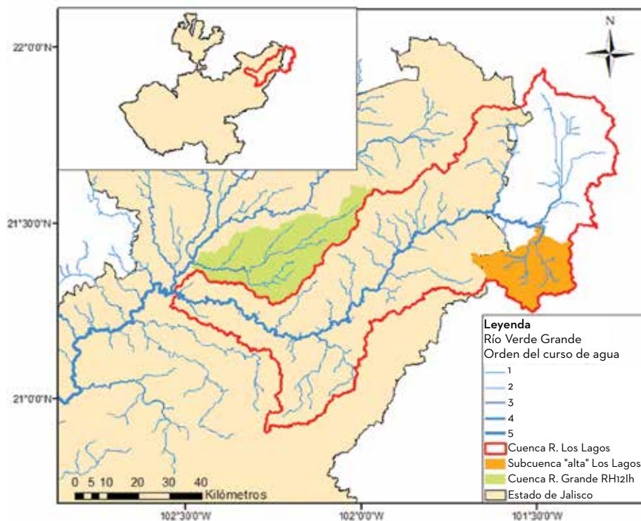
FIGURA 9.4 ZONAS REPRESENTATIVAS DE INTERÉS. ANÁLISIS GEOESPACIAL Y MULTITEMPORAL
