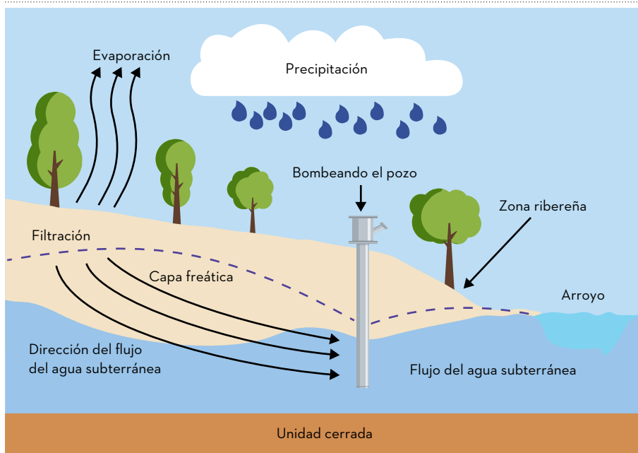
FIGURA 2.4 FLUJOS DEL AGUA SUBTERRÁNEA EN UN ACUÍFERO
