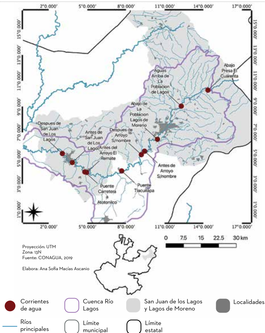
FIGURA 5.8 ESTACIONES DE MONITOREO DE CALIDAD DEL AGUA EN EL RÍO LAGOS
