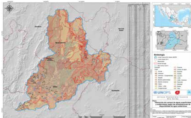
FIGURA 5.6 ZONAS DE RECARGA EN LA CUENCA DEL RÍO VERDE
