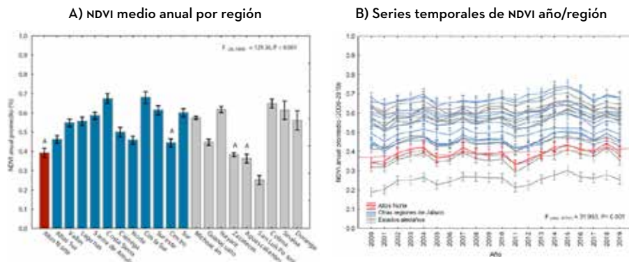
FIGURA 8.6 NDVI MEDIO ANUAL HISTÓRICO EN ALTOS NORTE Y SUS REGIONES DE INFLUENCIA, 2000-2019
