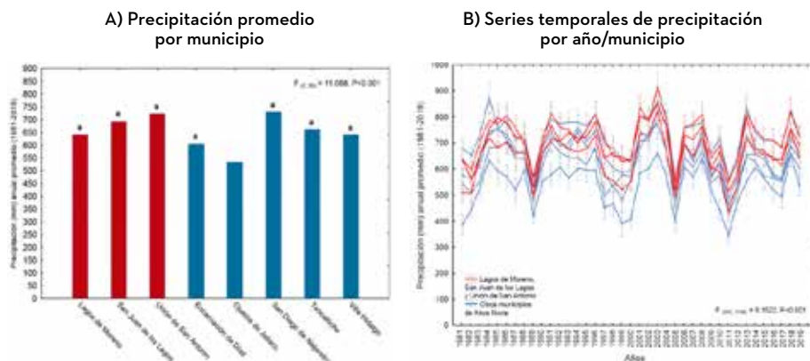
FIGURA 8.7 PRECIPITACIÓN MEDIA ANUAL HISTÓRICA DE LOS MUNICIPIOS DE LA REGIÓN ALTOS NORTE, 1981-2019
