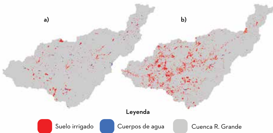
FIGURA 9.6 IMÁGENES CON CLASIFICACIÓN SUPERVISADA PARA LA SUBCUENCA DEL RÍO GRANDE, 1986 Y 2020
