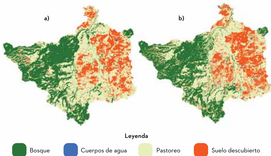
FIGURA 9.8 IMÁGENES CON CLASIFICACIÓN SUPERVISADA PARA LA SUBCUENCA ALTA DEL RÍO LAGOS, 1986-2020
