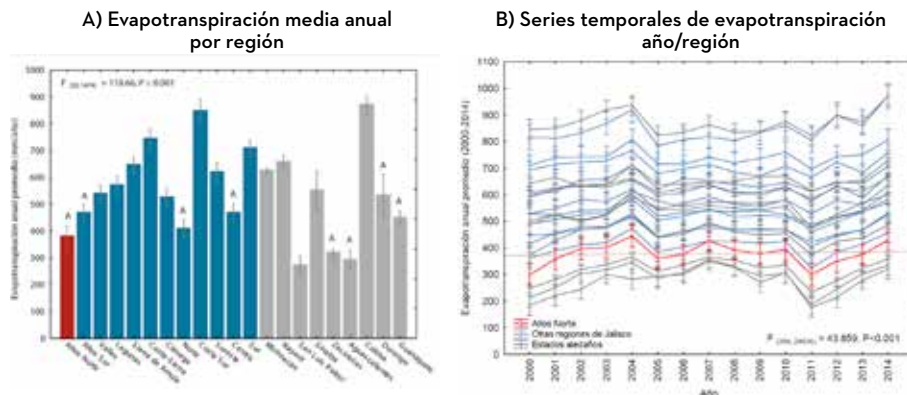
FIGURA 8.5 EVAPOTRANSPIRACIÓN MEDIA ANUAL HISTÓRICA EN ALTOS NORTE Y SUS REGIONES DE INFLUENCIA, 2000-2014
