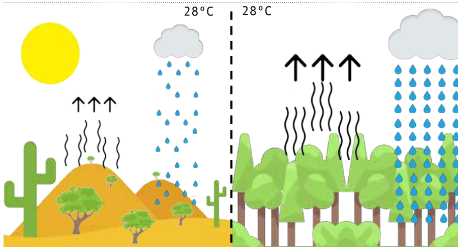
FIGURA 8.1 ESQUEMA DE LA RELACIÓN ENTRE TEMPERATURA, PRECIPITACIÓN, EVAPOTRANSPIRACIÓN Y VEGETACIÓN
