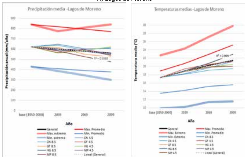
FIGURA 9.1. PRECIPITACIÓN ANUAL Y TEMPERATURA MEDIA ANUAL PARA TRES MUNICIPIOS DE LA REGIÓN ALTOS NORTE DE JALISCO
